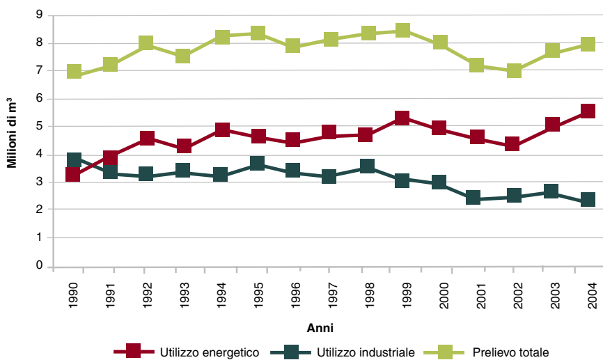
Grafico 2 - Evoluzione e dei prelievi legnosi (per fini energetici e industriali) da foresta in Italia (1990-2004).
